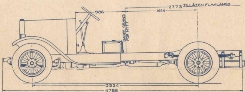
LV-60 "1 \frac{1}{2} ton" Hjulbas 3324 mm. Kr. 4975:—
