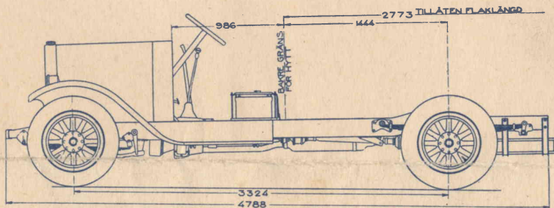
LV-62 "2 ton" Hjulbas 3324 mm.
