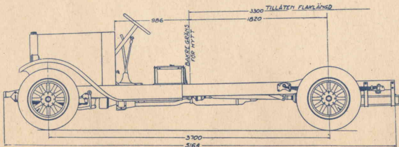
LV-61 "1 \frac{1}{2} ton" Hjulbas 3700 mm. Kr. 5150:—
