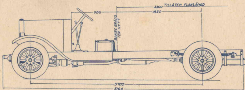
LV-63 "2 ton" Hjulbas 3700 mm.
